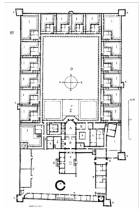
Planta tipo de monasterio cartujano, Clermont, dibujada por Eugène Viollet-le-Duc, 1856.
